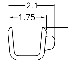
Section D-D
