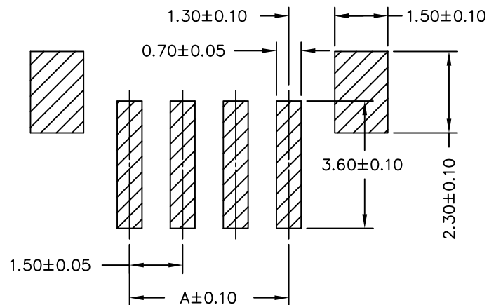
P.C.B LAYOUT
